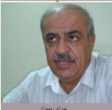
نەوزاد رەمەزان
